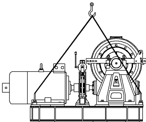
吊装示意图(YJ410)
