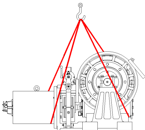
吊装示意图(YJ240B、YJ275、YJ320)
