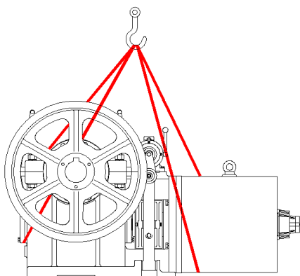
吊装示意图(FYJ180、FYJ200、FYJ245)
