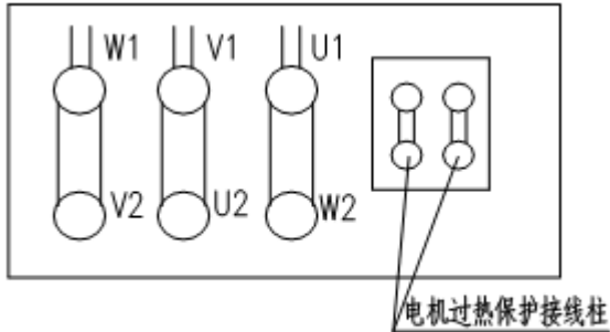
电机接线板示意图
