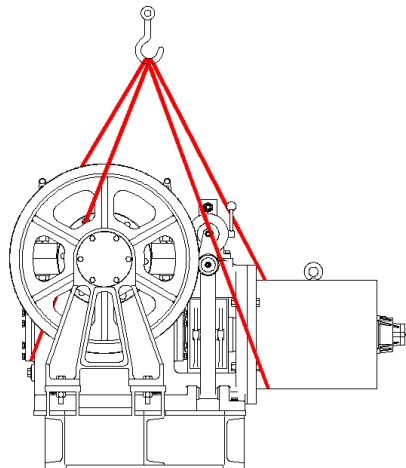
吊装示意图(YJ200、YJ245D)
