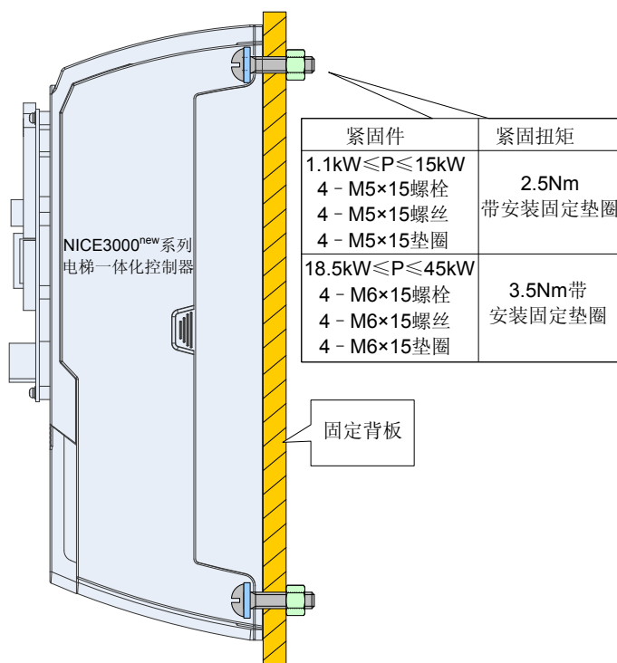
图 3-2 安装孔位紧固示意图
