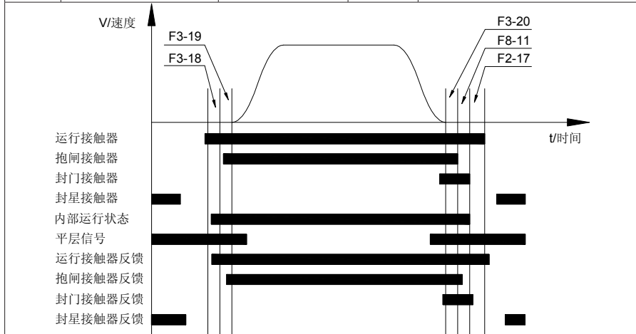
图 5-4 运行时序图
