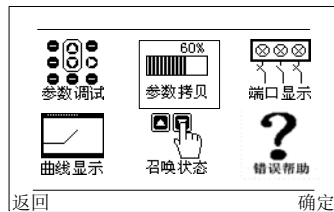
图 4-12 液晶操作器主界面
