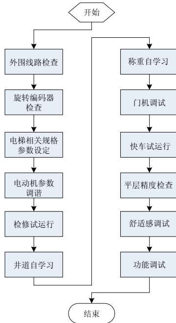
图 5-1 NICE3000 new 系列一体化控制器系统调试流程
