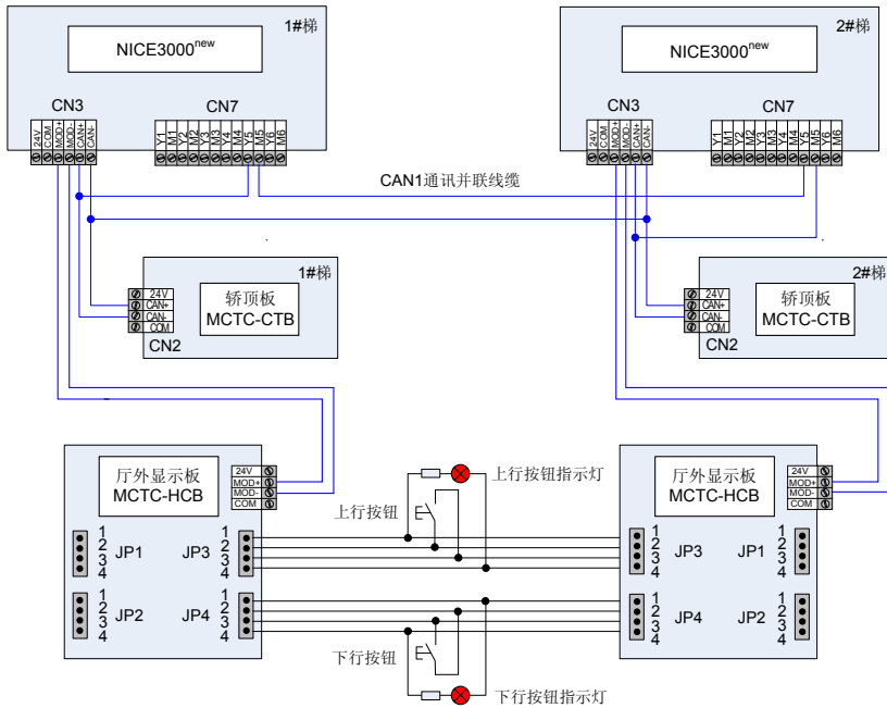
图 5-11 使用 CAN1 通讯并连接示意图
