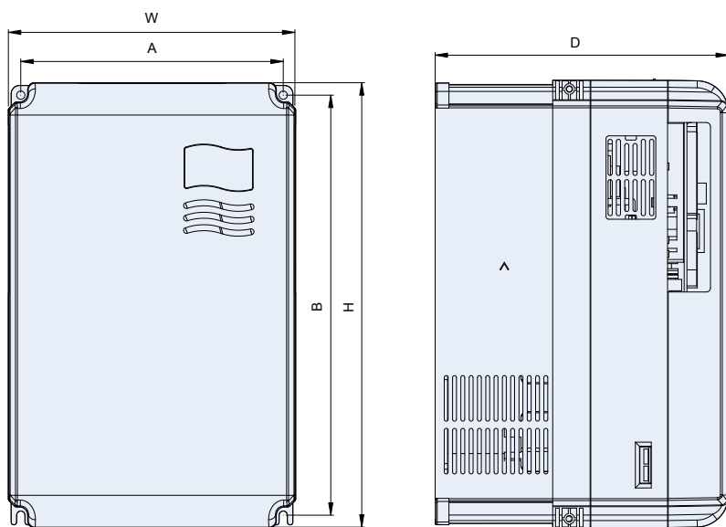
图 2-6 L1 结构尺寸示意图
