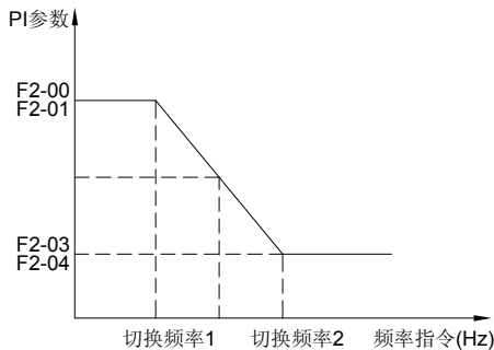
图 7-1 PI 参数示意图
