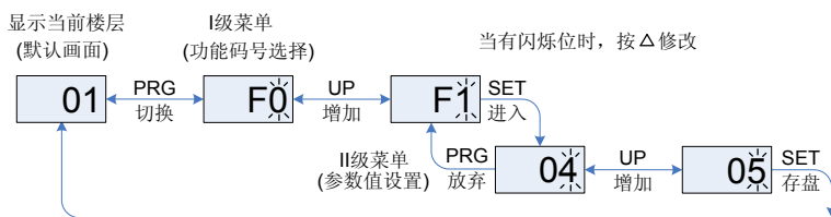
图 4-2 呼梯设定过程
