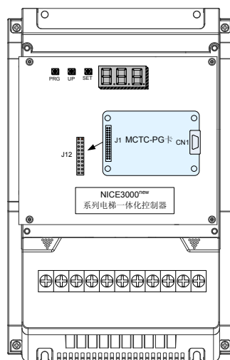
图 3-14 MCTC-PG 卡实物及安装示意图
