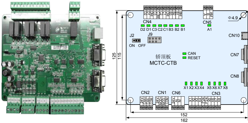
图 3-6 轿顶板外观及尺寸 (单位: mm)
