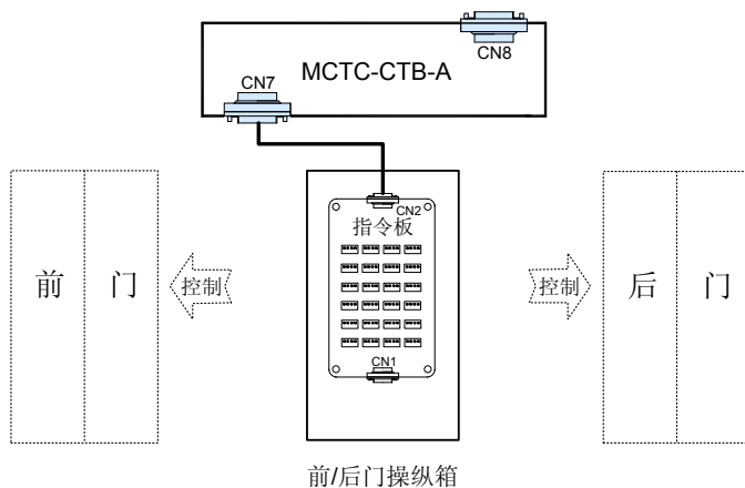
图 5-13 控制模式 1、2、3 轿内指令板接线图（单操纵箱）
