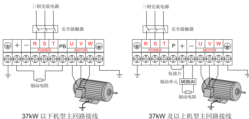
图 3-5 主回路接线示意图
