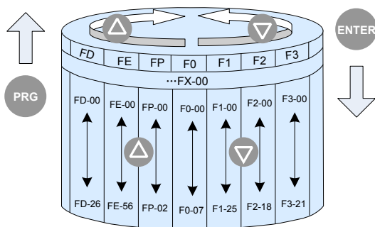
图 4-5 三级菜单切换关系示意图
